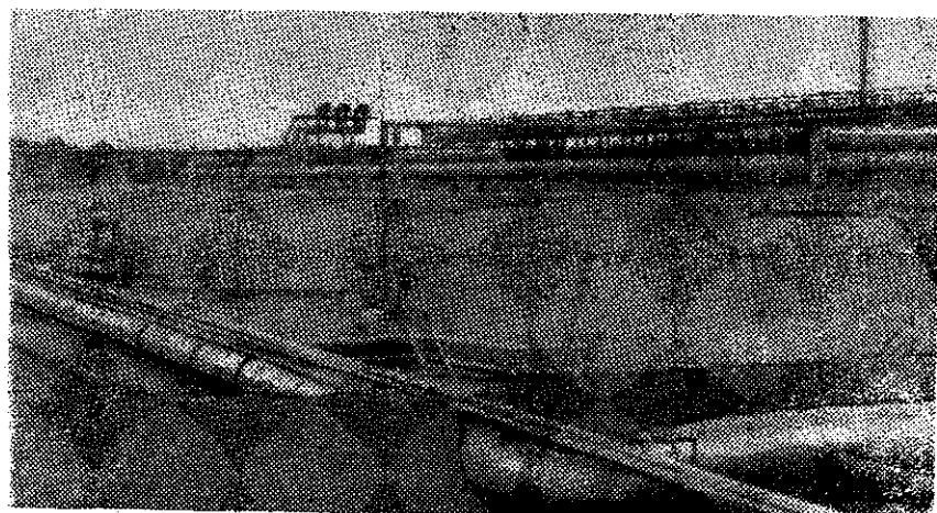
Кирпичный Нефтеперерабатывающий завод. Парк смешения нефти, сданный в эксплуатацию строителями 25-го управления. Фото В. Приотина.
