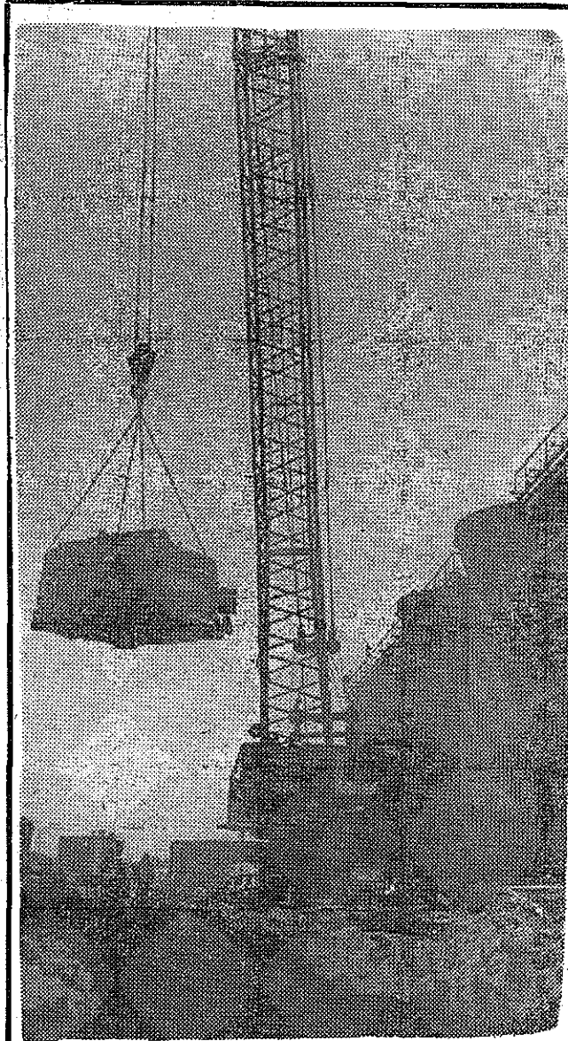
Водоблок обратного водоснабжения — один из важных объектов комплекса атмосферно-вакуумной трубчатки на Киришском нефтеперерабатывающем заводе. Сейчас на водоблоке идут завершающие работы. В конце года он будет предъявлен заказчику. Фото В. Приотина.
